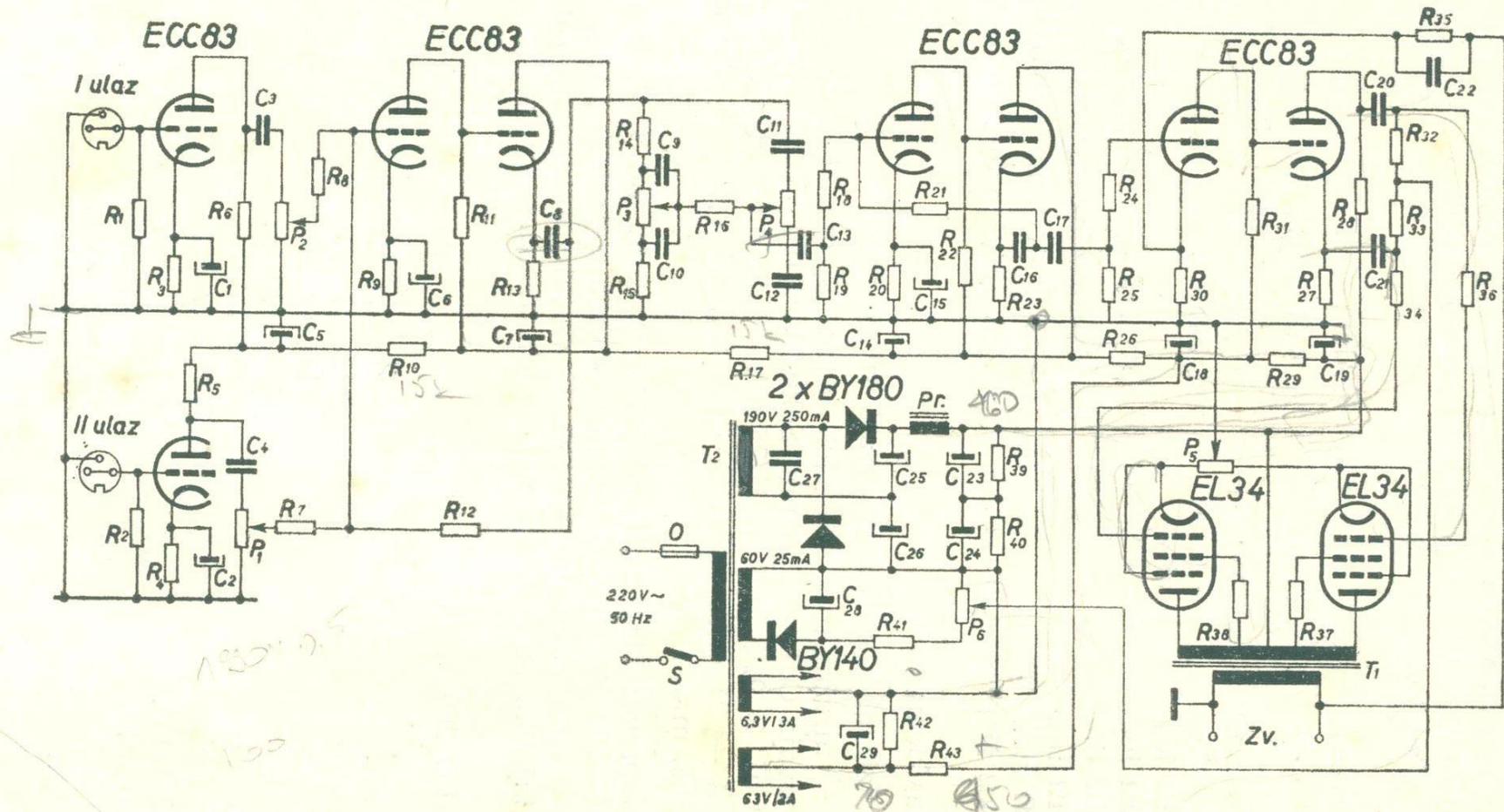
Sl. 68 — Hi-Fi pojačalo od 55 W za bas gitaru
